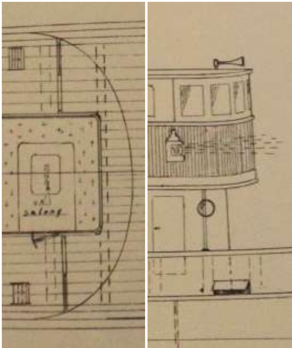
figur 19: overbygg forut som planlagt i GA-tegninger, 1943 (utsnitt av figur 116).
